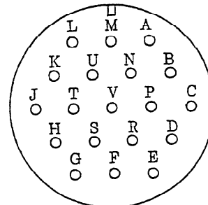
MS3102A22-14P
