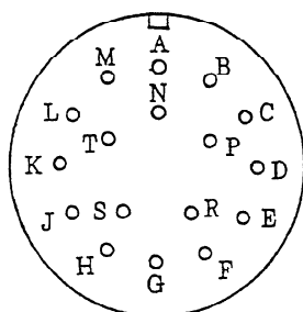
MS3102A20-29P
