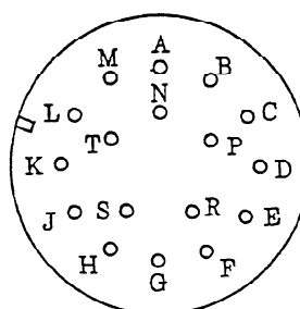
MS3102A20-29PW
